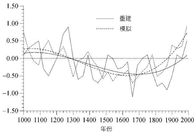
图 3 1000 年来中国东部温度距平变化的模拟与重建对比
