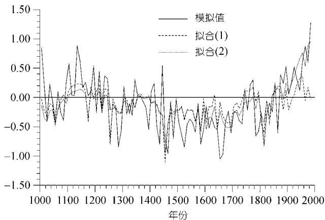
图4 模拟的中国东部温度距平及其拟合曲线
