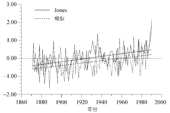
图2 中国东部区域冬半年温度距平变化的模拟与 Jones 观测集成资料的对比
