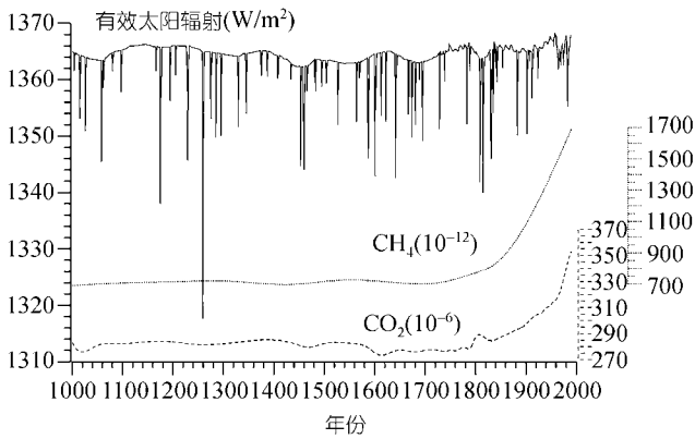
图1 强迫因子的时间变化
